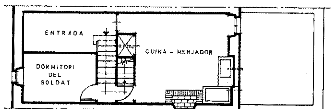
PLANTA ENTRESOL
