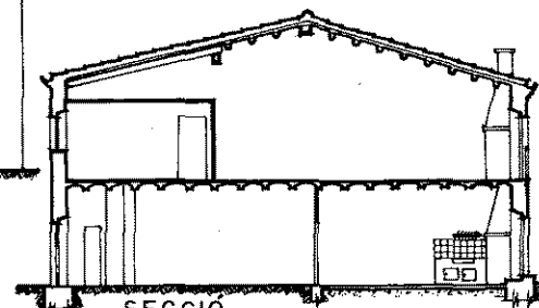
SECCIÓ
