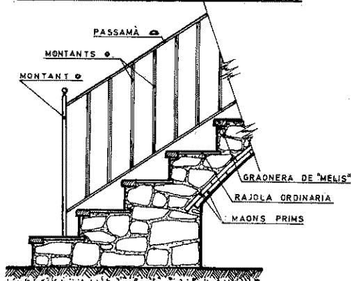
SECCIÓ ESCALA - Barana de ferro
