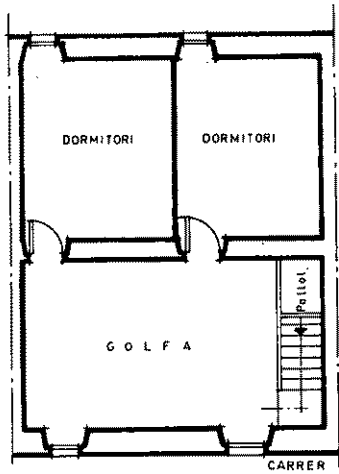
PLANTA GOLFES
