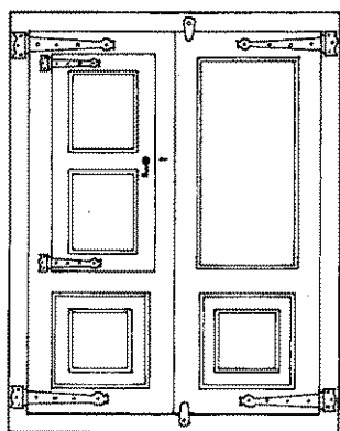
Alçat interior
