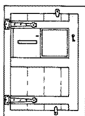
Alçat interior
