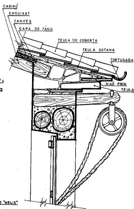
SECCIÓ DE BARBACANA I TEULADA
