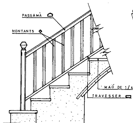
ALÇAT ESCALA - Barana de fusta
