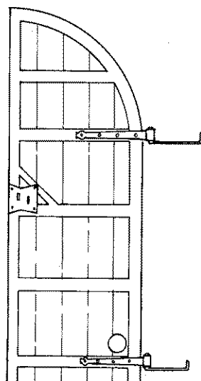
Alçat interior
