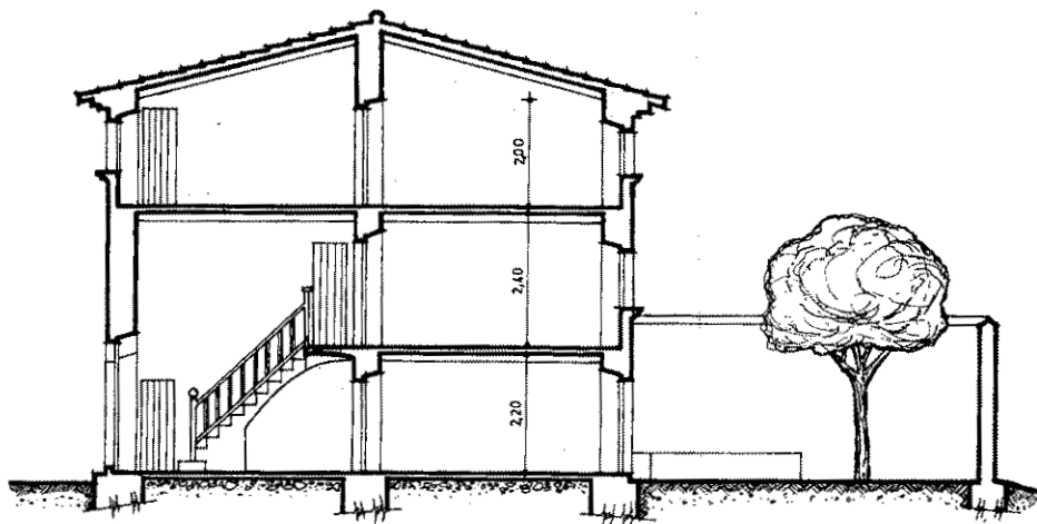
SECCIÓ LONGITUDINAL
