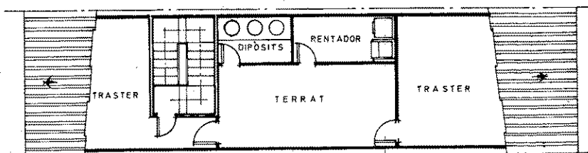
PLANTA COBERTA
