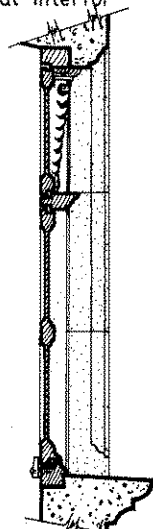
Secció
