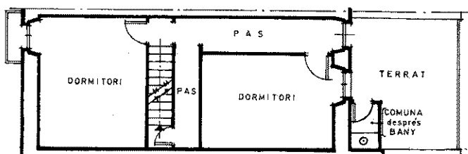
PLANTA PRINCIPAL
