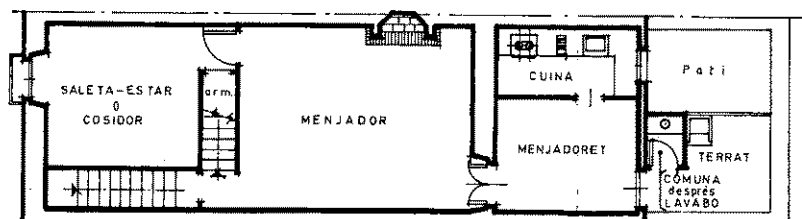
PLANTA ENTRESOL
