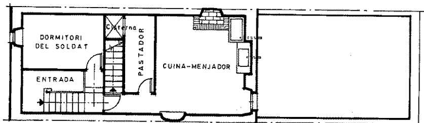
PLANTA ENTRESOL
