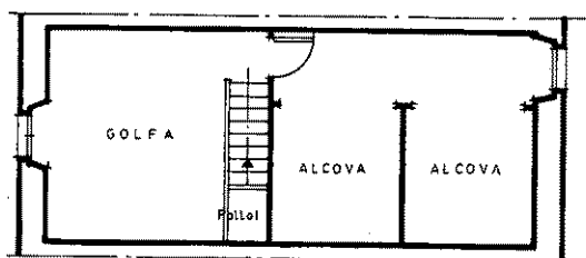
PLANTA GOLFES
