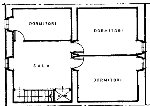
PLANTA PRINCIPAL
