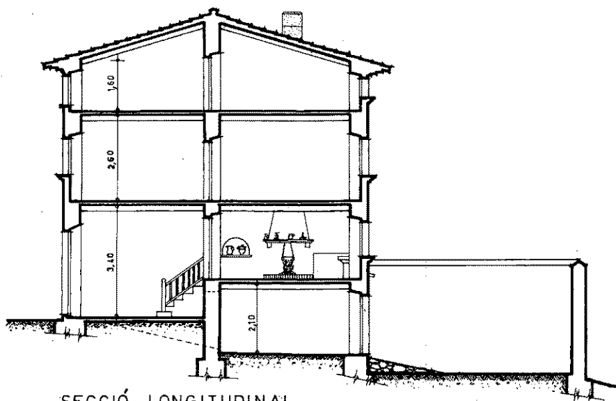
SECCIÓ LONGITUDINAL
