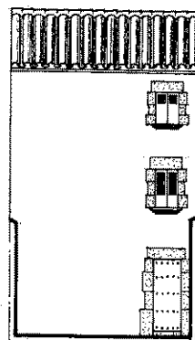
FAÇANA POSTERIOR
