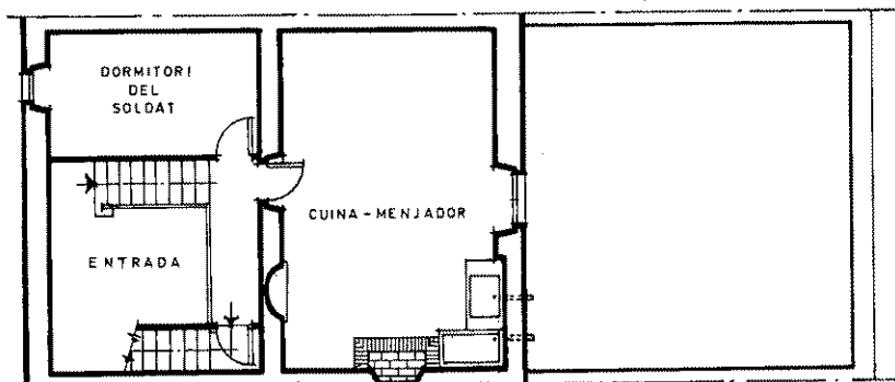
PLANTA ENTRESOL
