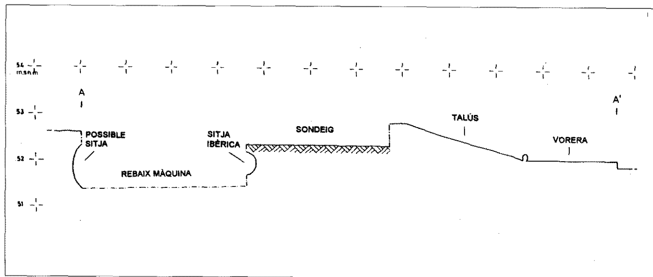
Figura 3: Secció en sentit oest - est de l'àrea de la intervenció arqueològica (plànol extret de Codex 1998).
