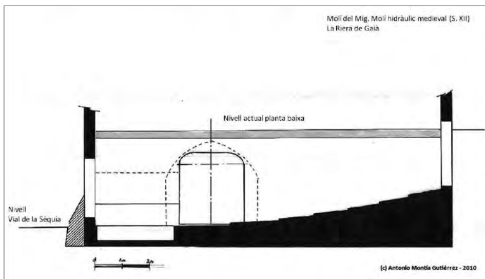
Molí del Mig – secció longitudinal
