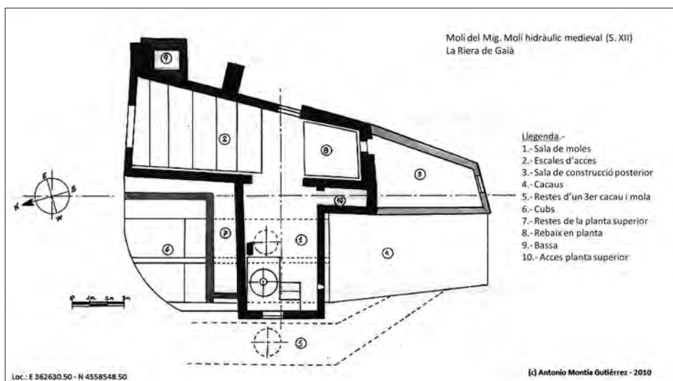
Molí del Mig – planta
