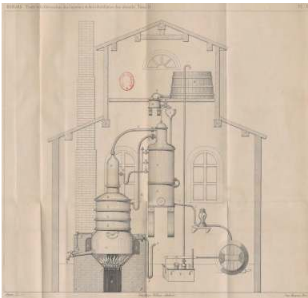
Gravat d'un alambí industrial, a les planxes al final del llibre Traité de la fabrication des liqueurs et de la distillation des alcools... , de P. Duplais, de 1867, de la Bibliothèque Nationale de France (BNF, Gallica )
