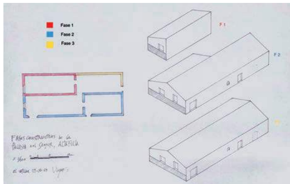
Fig. 7. Esquema en planta i bloc-diagrama de les fases constructives.
