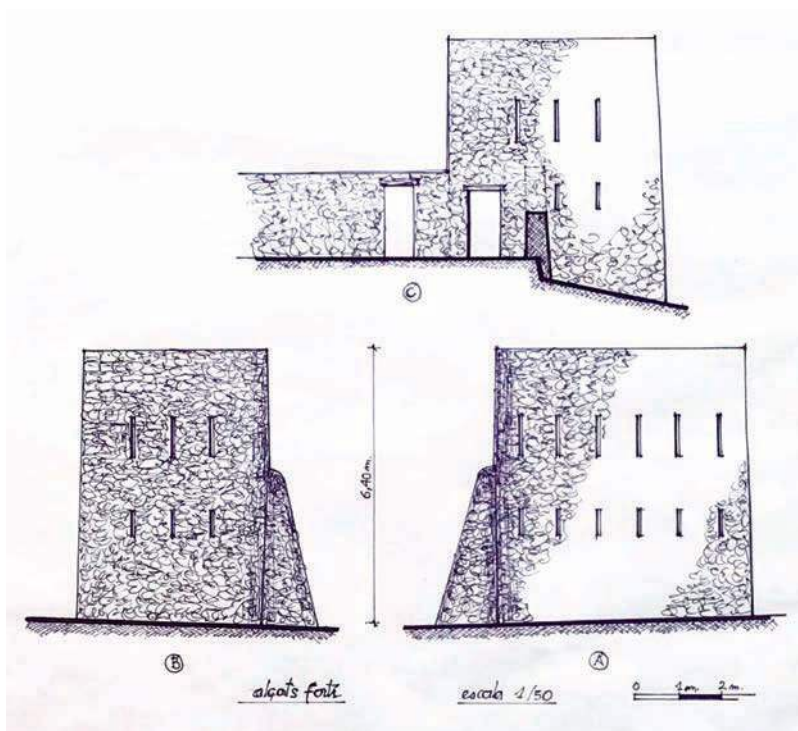
Figura 4. Façanes de la torre, amb el contrafort i dues files d'espitlleres.
