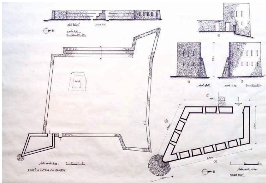
Figura 2. Planta i seccions del conjunt del fortí.
