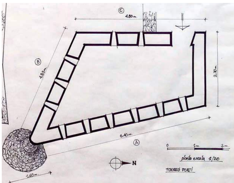
Figura 5. Planta de la torre del fortí amb les espitlleres situades als tres murs, excepte al nord, defensat pel baluard annex.
